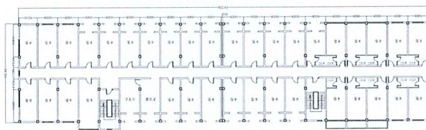
宿舍楼 二~五层平面图
