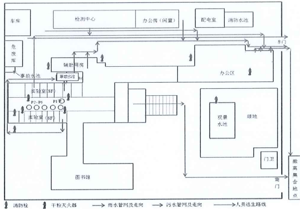
海洋化工研究院本部平面布局图
