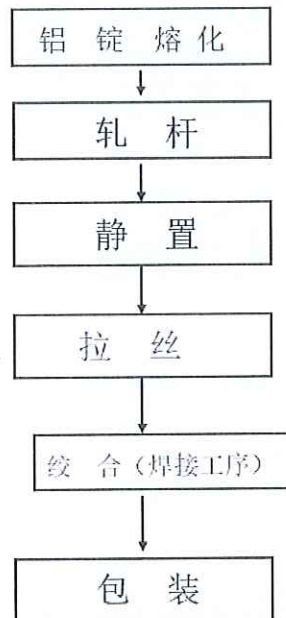
铝绞线工艺流程图
