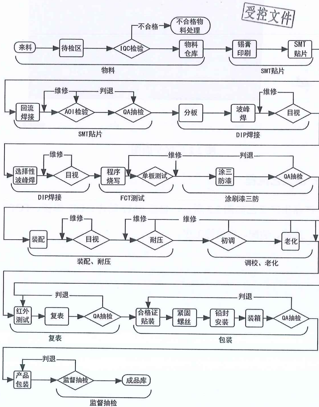
图 2.3 单相费控智能电能表 (DDZY193-M) 工艺流程图
