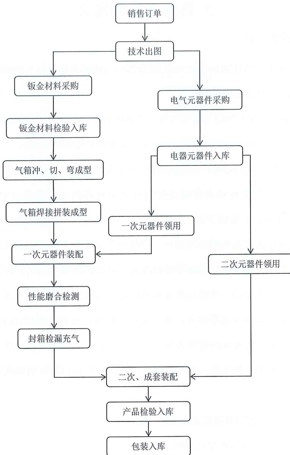
图 2.3 全绝缘全密封金属封闭环网开关设备（VEJS-12V/T630-
