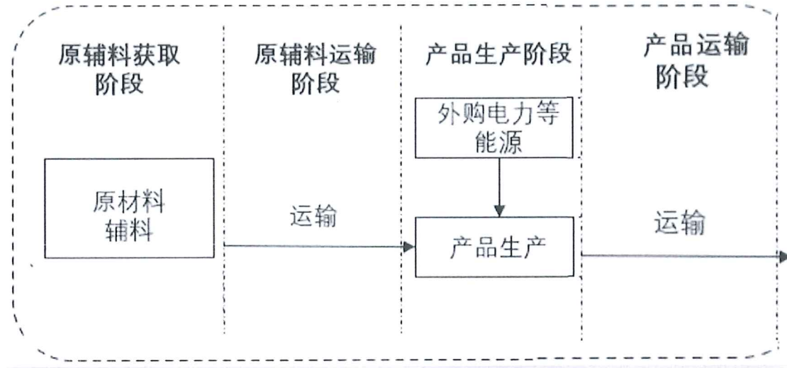
图 3.1: 系统边界
