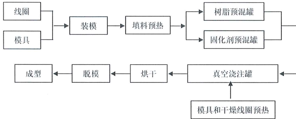
图 3-1 全真空浇注生产工艺流程图
