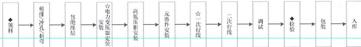
箱式变电站实现过程流程图
