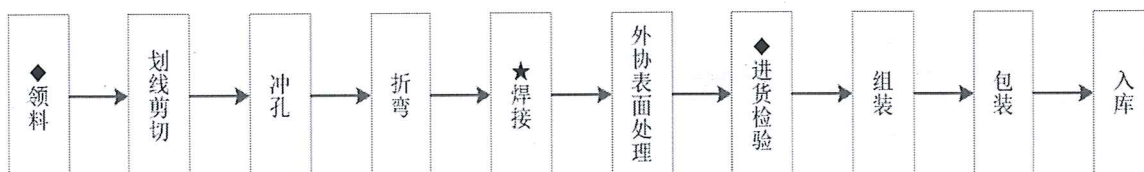
高低压柜壳体实现过程流程图
