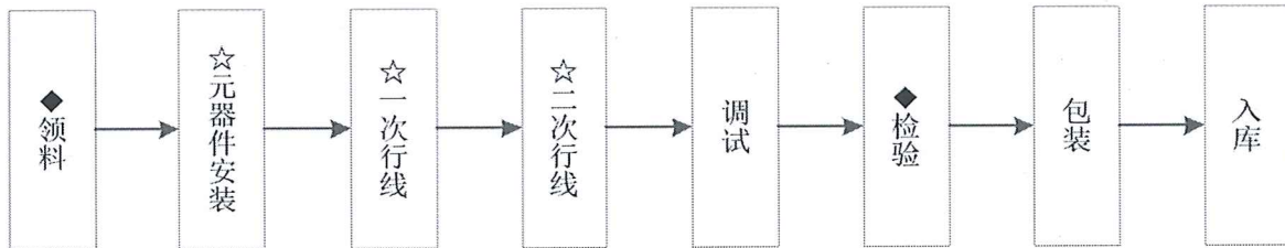
高低压成套开关设备实现过程流程图
