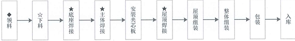
箱变壳体实现过程流程图
