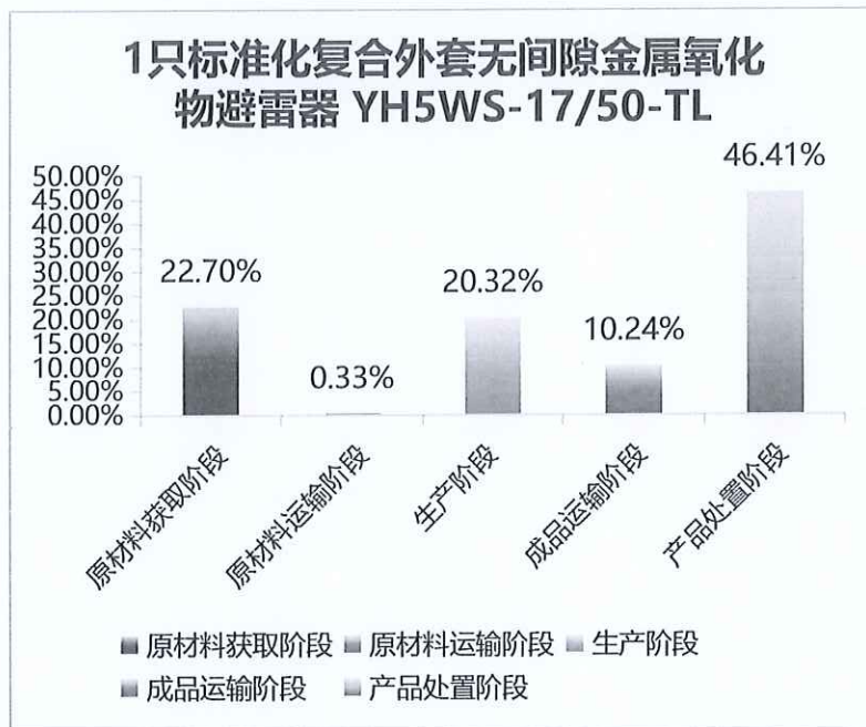
图 5.2-2 一只标准化复合外套无间隙金属氧化物避雷器（YH5WS-17/50-TL）生命周期阶段碳排放分布图
