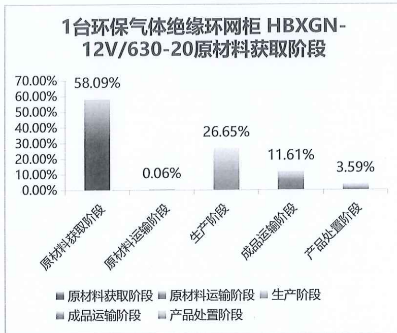
图 5.2-2 一台环保气体绝缘环网柜（HBXGN-12V/630-20）生命周期阶段碳排放分布图
