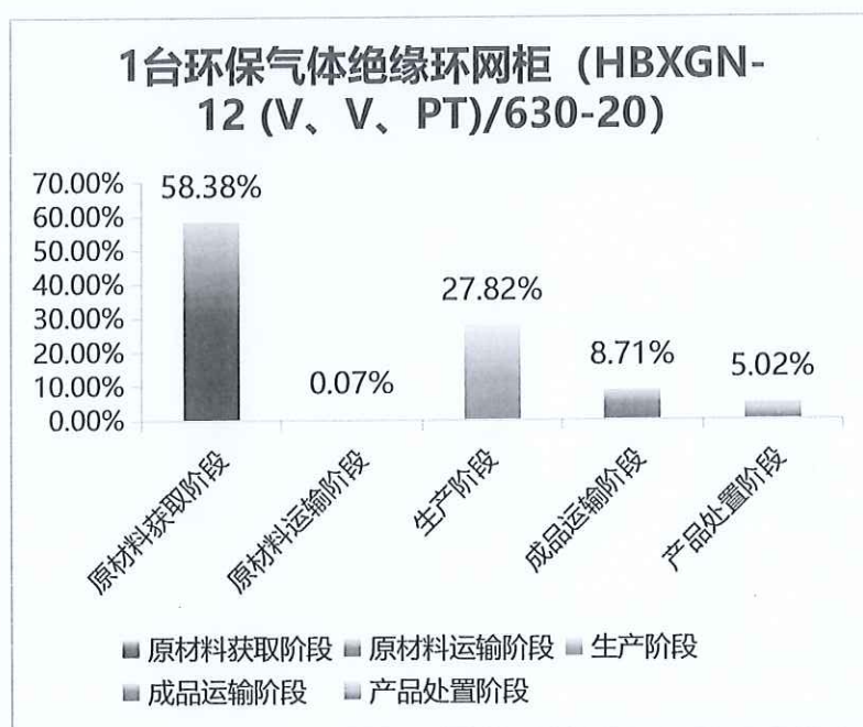
图 5.2-2 一台环保气体绝缘环网柜 (HBXGN-12 (V、V、PT)/630-20) 生命周期阶段碳排放分布图
