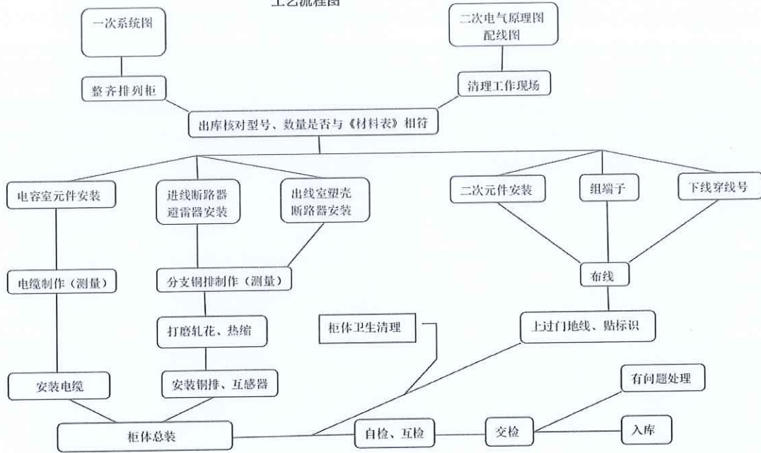
工艺流程图
