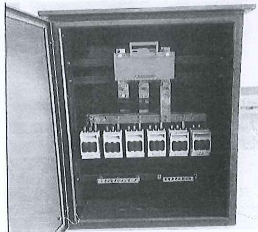
内部结构
