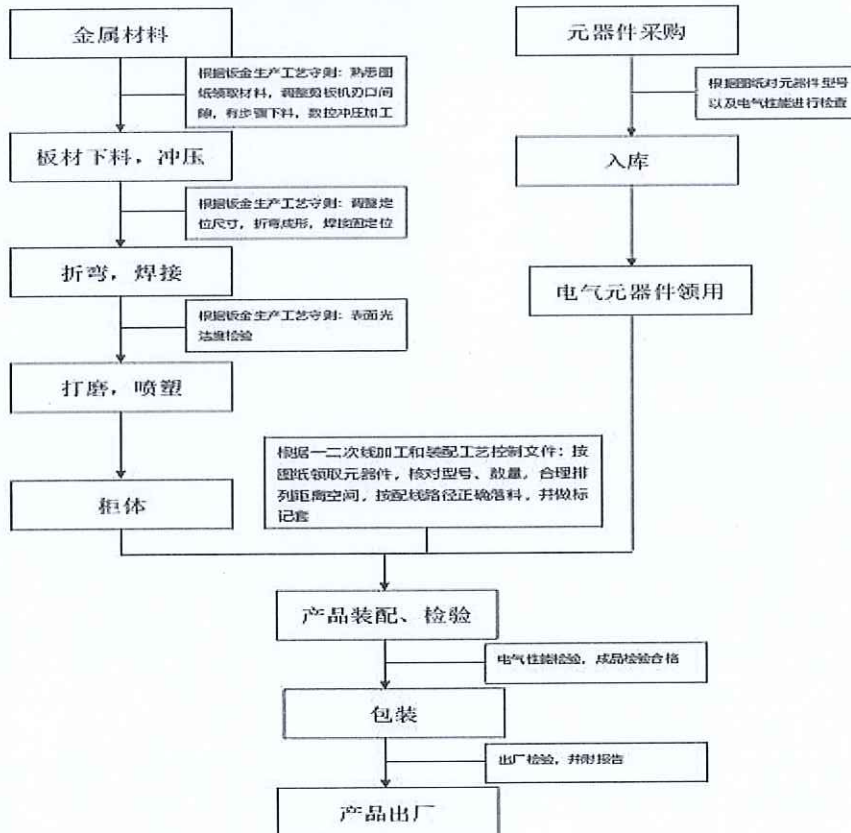
高低压电缆分支箱工艺流程
