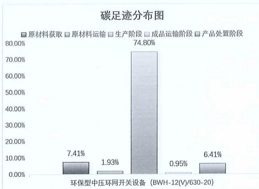
图 5.2.1.2 环保型中压环网开关设备 (BWH-12(V)/630-20) 生命周期阶段碳排放分布图
