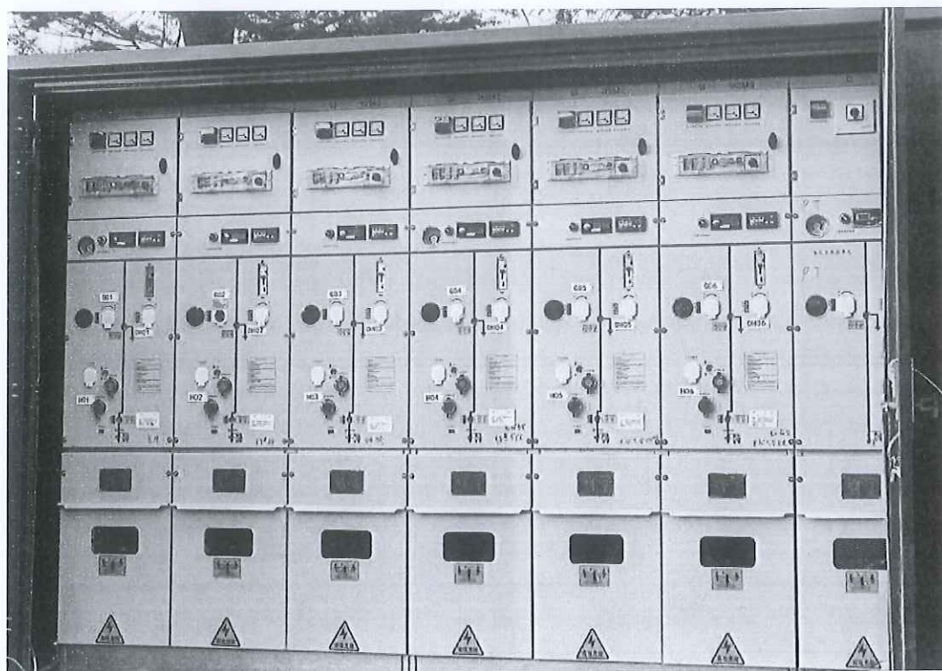
环保型中压环网开关设备 (BWH-12(V)/630-20)
