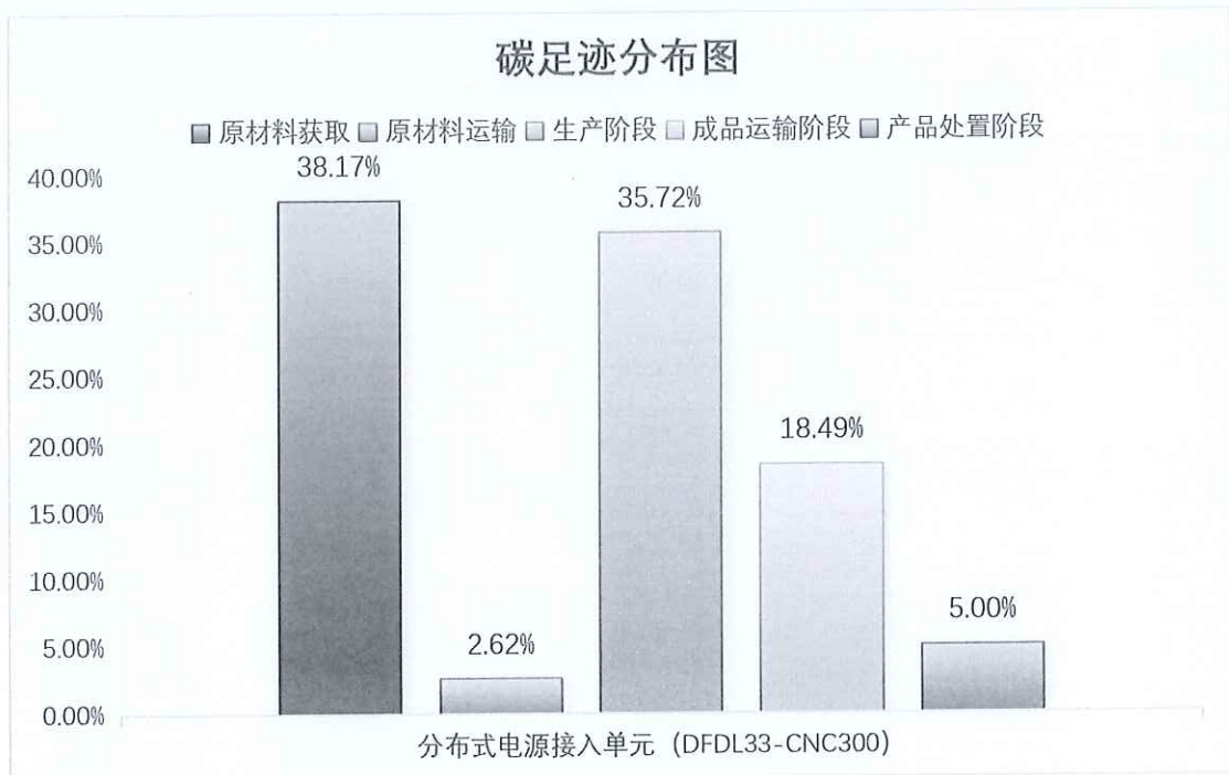
图 5.2.1.2 分布式电源接入单元 (DFDL33-CNC300) 生命周期阶段碳排放分布图
