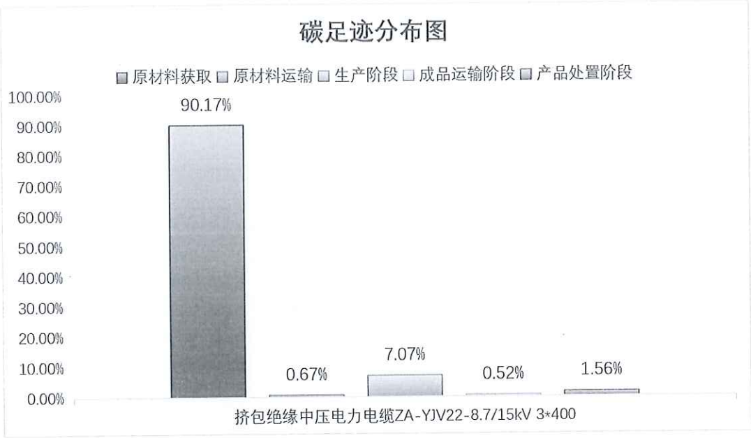
图 5.2.2-2 产品生命周期阶段碳排放分布图
