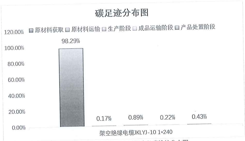
图5.2.3-2 产品生命周期阶段碳排放分布图
