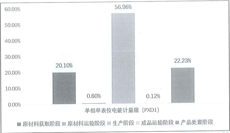
图 5.2-2-3 1 台单相单表位电能计量箱（PXD1）生命周期阶段碳排放分布图
