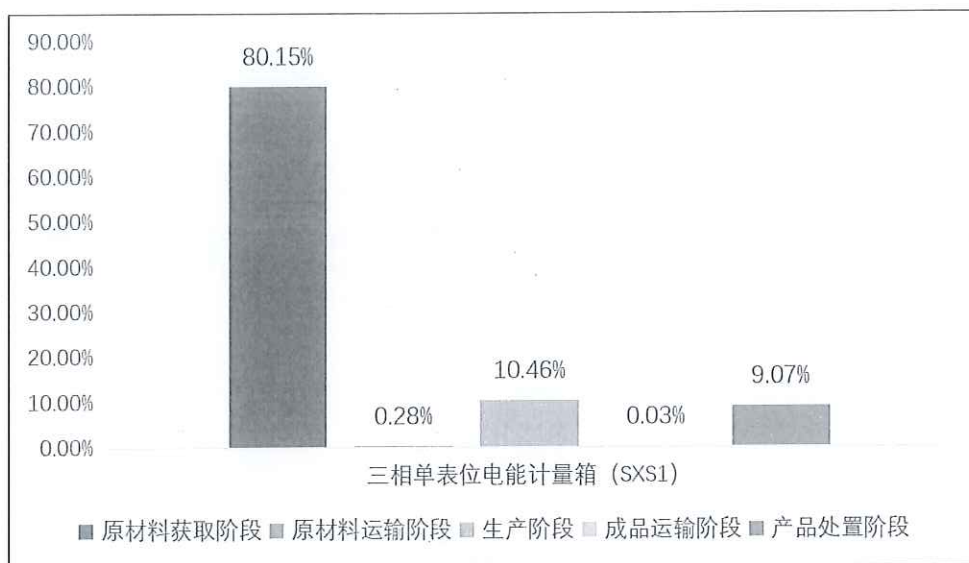
图 5.2-2-8 1 台三相单表位电能计量箱 (SXS1) 生命周期阶段碳排放分布图
