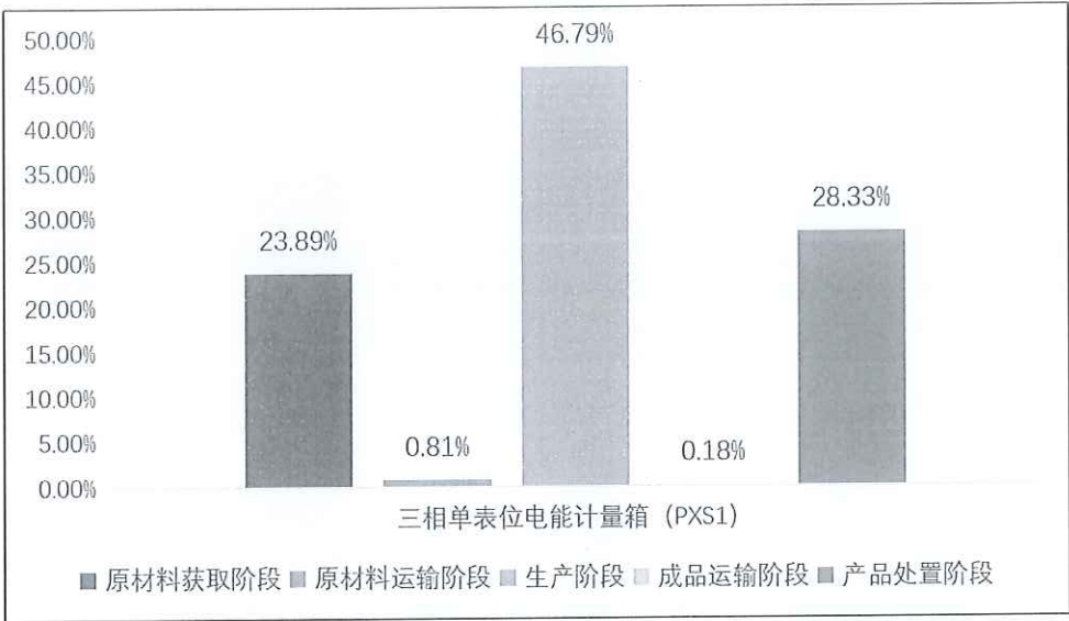
图 5.2-2-5 1 台三相单表位电能计量箱 (PXS1) 生命周期阶段碳排放分布图
