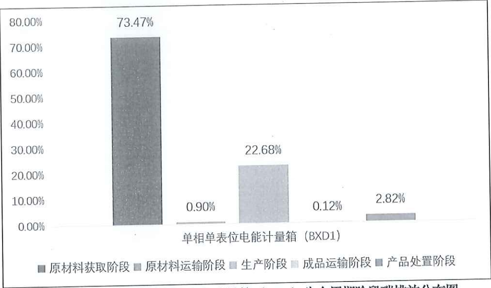
图 5.2-2-1 1 台单相单表位电能计量箱（BXD1）生命周期阶段碳排放分布图
