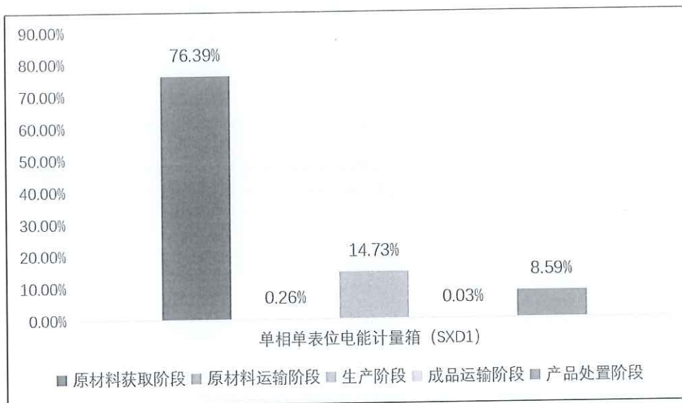
图 5.2-2-7 1 台单相单表位电能计量箱 (SXD1) 生命周期阶段碳排放分布图
