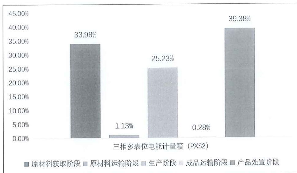
图 5.2-2-6 1 台三相多表位电能计量箱 (PXS2) 生命周期阶段碳排放分布图
