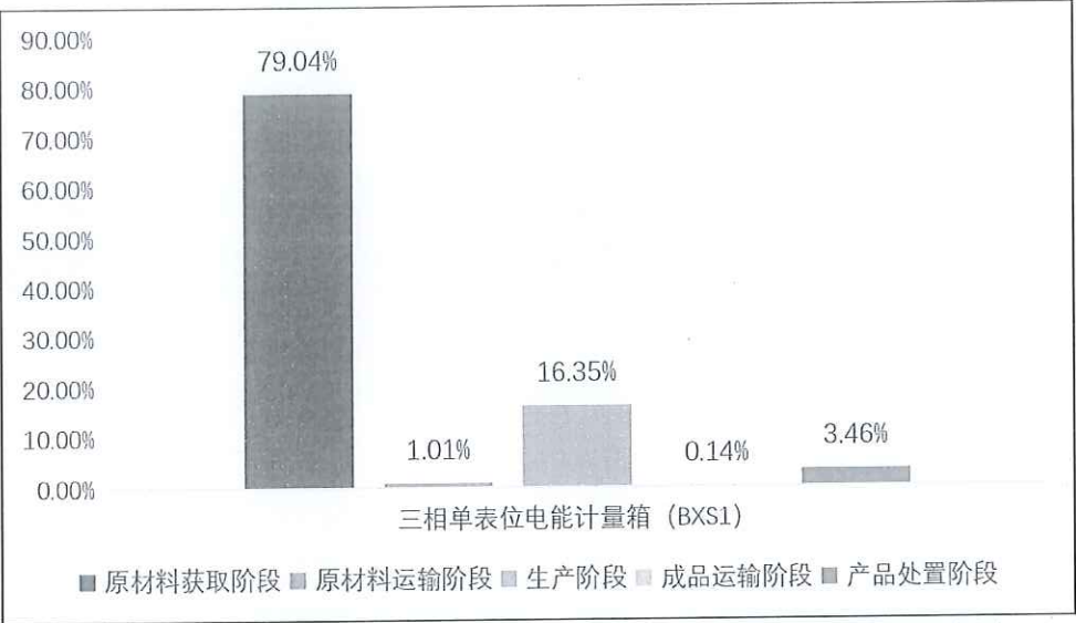
图 5.2-2-2 1 台三相单表位电能计量箱（BXS1）生命周期阶段碳排放分布图
