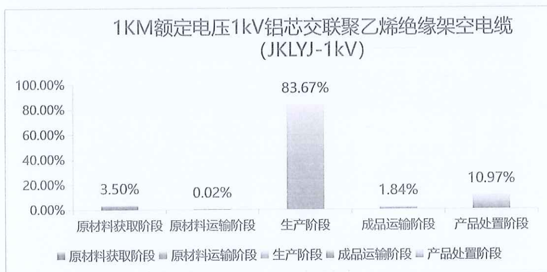
图 5.2-2 1KM 额定电压 1kV 铝芯交联聚乙烯绝缘架空电缆（JKLYJ-1kV）生命周期阶段碳排放分布图
