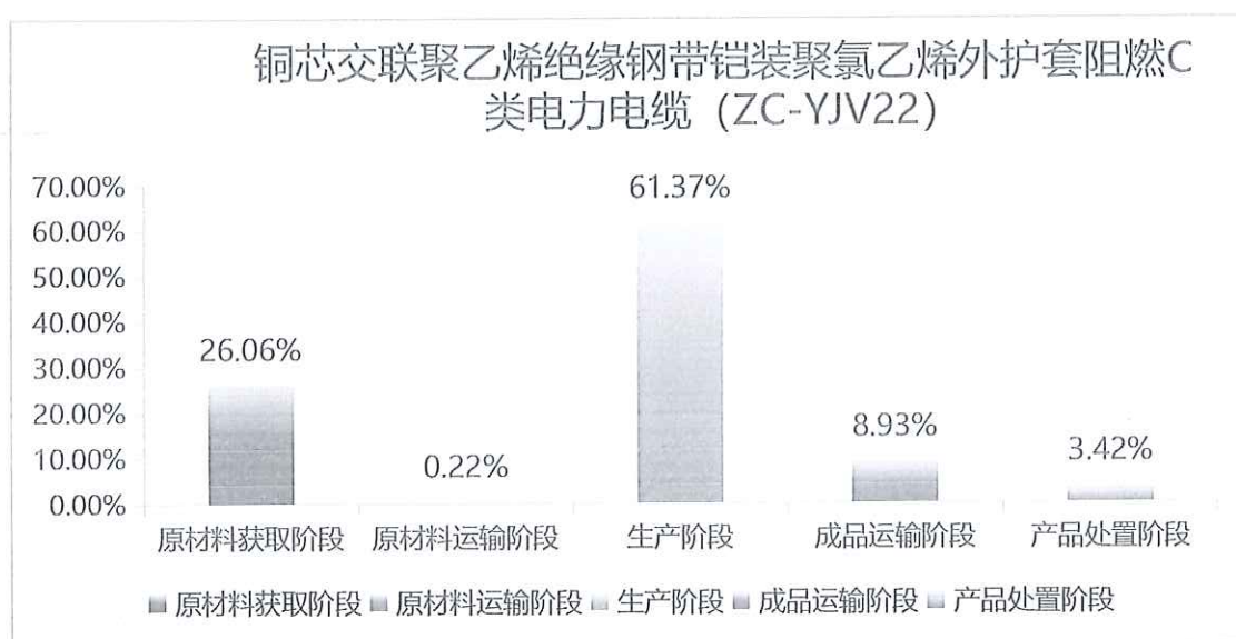
图 5.2-2 1KM 铜芯交联聚乙烯绝缘钢带铠装聚氯乙烯外护套阻燃 C 类电力电缆（ZC-YJV22）生命周期阶段碳排放分布图
