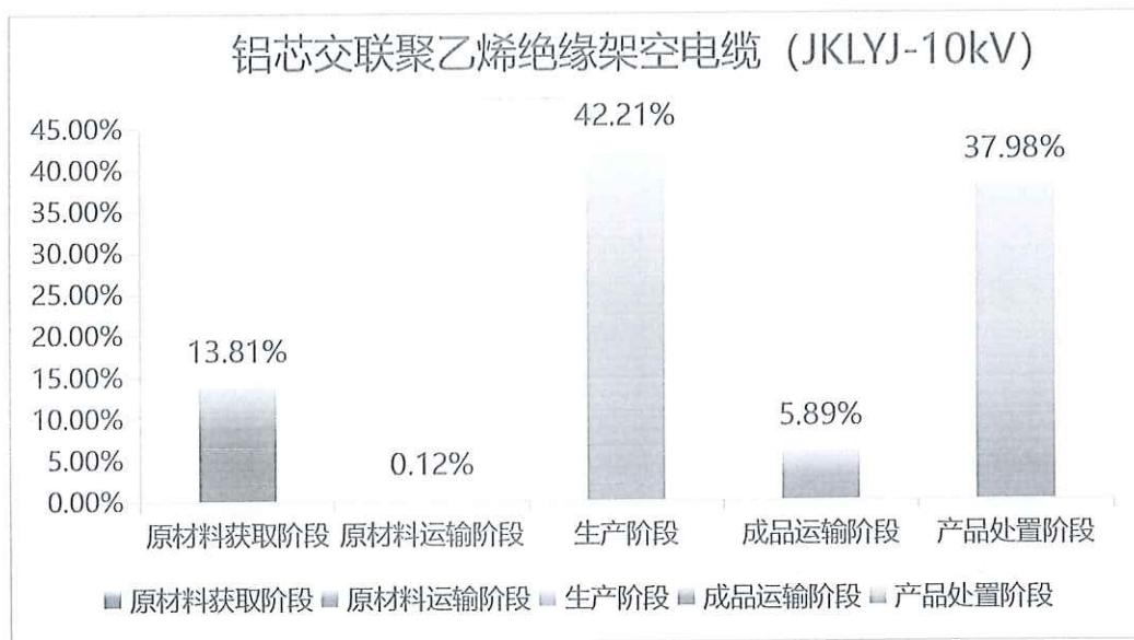
图 5.2-2 1KM 铝芯交联聚乙烯绝缘架空电缆（JKLYJ-10kV）生命周期阶段碳排放分布图
