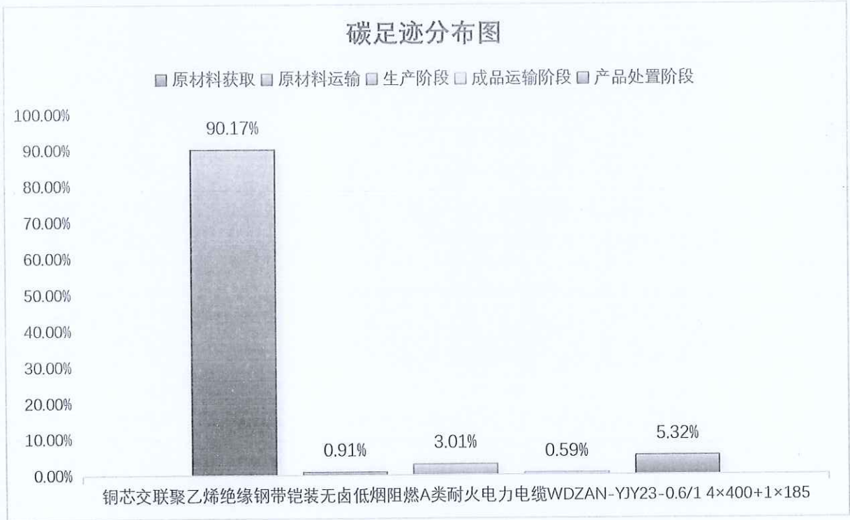
图 5.2.2-2 产品生命周期阶段碳排放分布图
