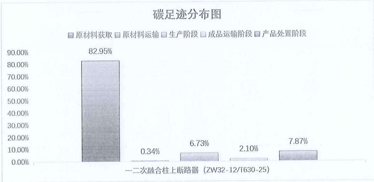
图 5.2-2 1 台一二次融合柱上断路器（ZW32-12/T630-25） 产品生命周期阶段碳排放分布图
