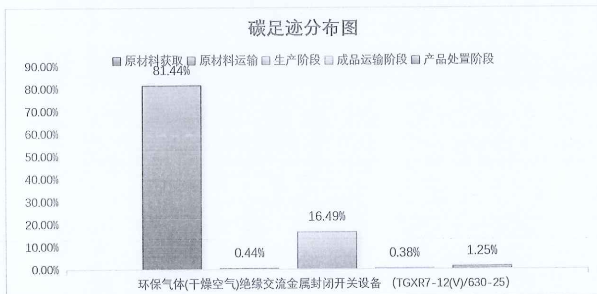
图 5.2-2 1 台环保气体(干燥空气)绝缘交流金属封闭开关设备（TGXR7-12(V)/630-25） 产品生命周期阶段碳排放分布图
