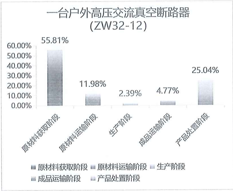
图 5.2-2 一台户外高压交流真空断路器（ZW32-12）生命周期阶段碳排放分布图
