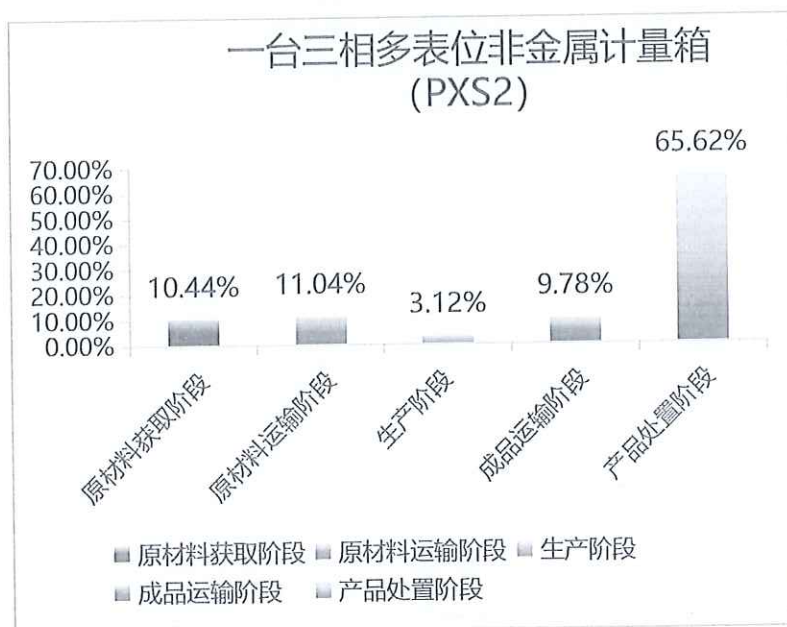
图 5.2-2 一台三相多表位非金属计量箱（PXS2）生命周期阶段碳排放分布图
