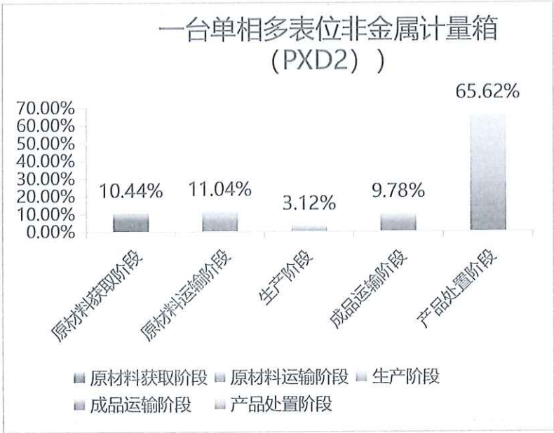
图 5.2-2 一台单相多表位非金属计量箱（PXD2）生命周期阶段碳排放分布图
