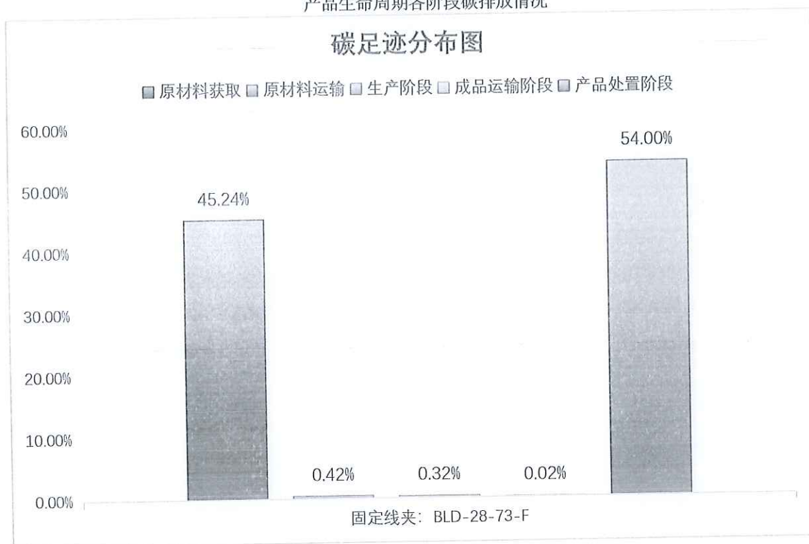
图 5.2-2 1 吨固定线夹（BLD-28-73-F） 产品生命周期阶段碳排放分布图
