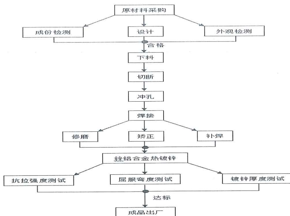
铁附件生产工艺流程图
