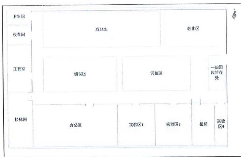
附图三 项目平面布局图(车间2层)
