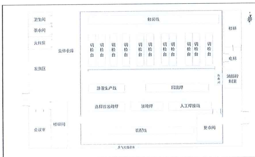
附图三 项目平面布局图(车间1层)
