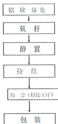
铝绞线工艺流程图
