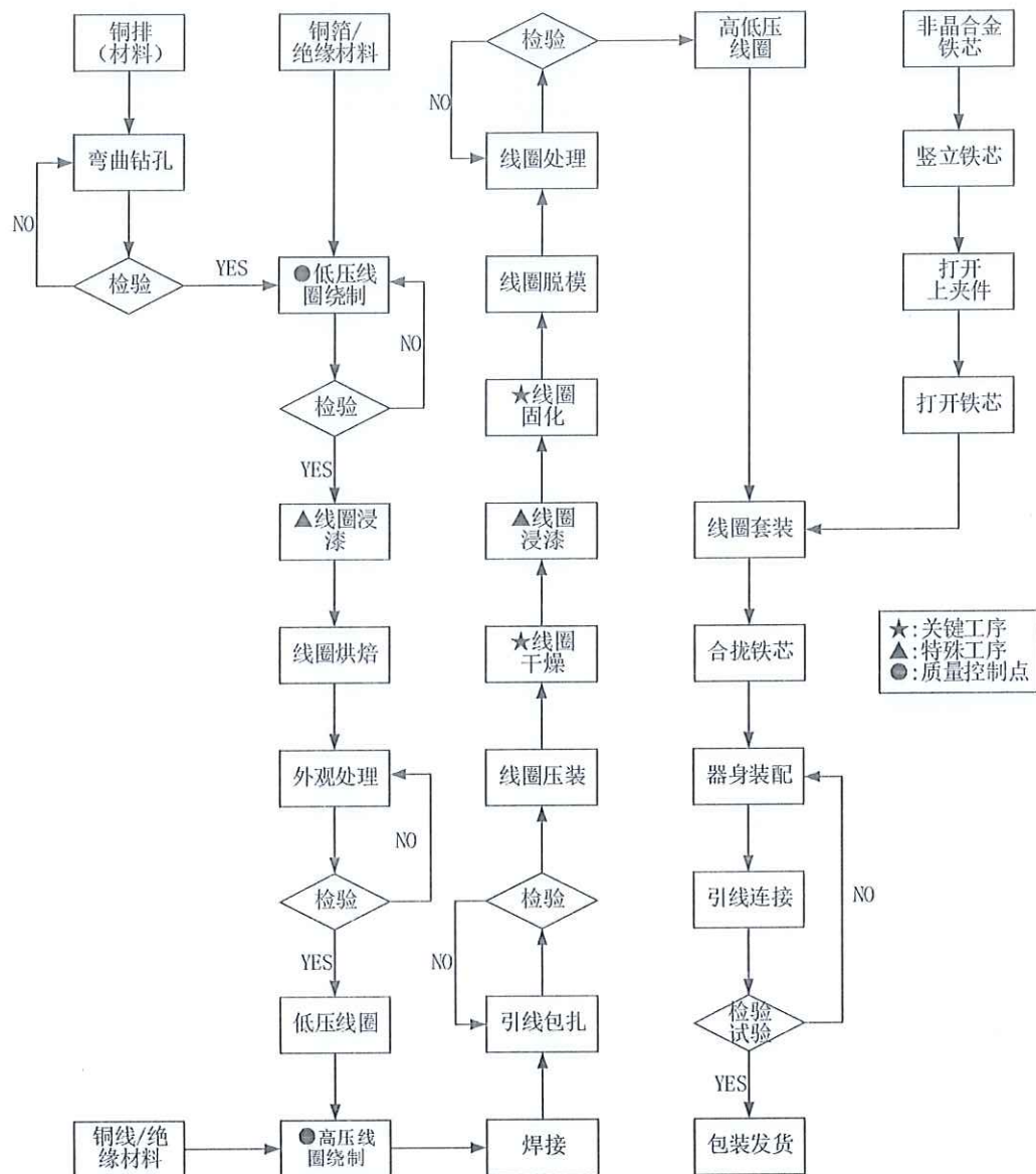
(2) 非晶合金干式变压器生产工艺流程图
