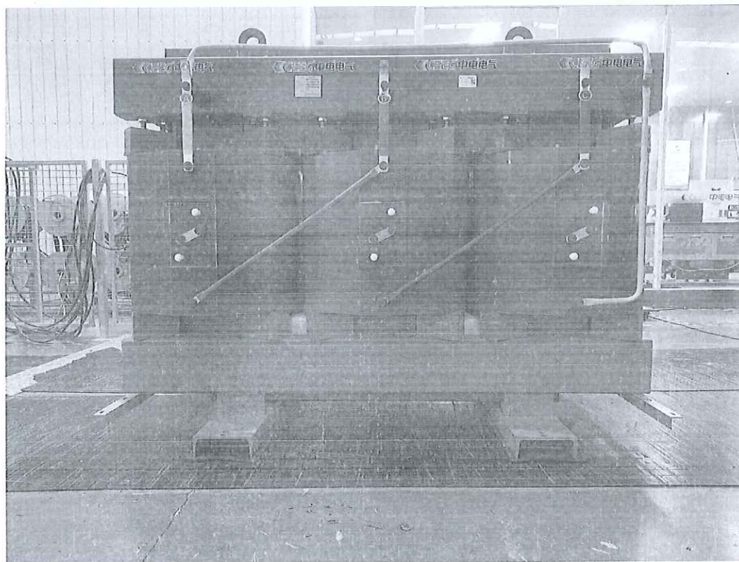
SCBH19 非晶合金变压器实拍图
