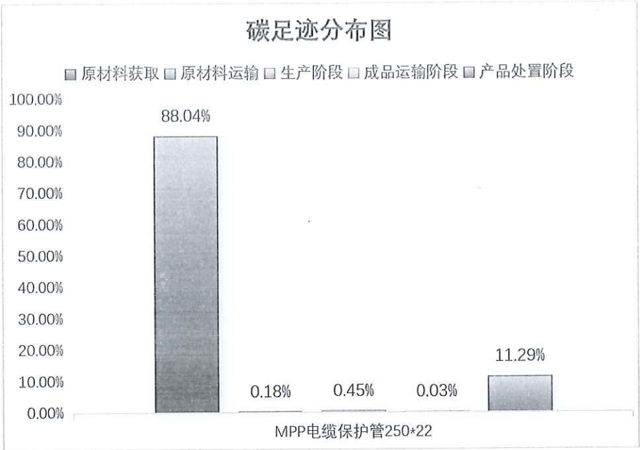
图 5.2.2-2 产品生命周期阶段碳排放分布图
