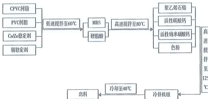
图1 混料工艺流程图
