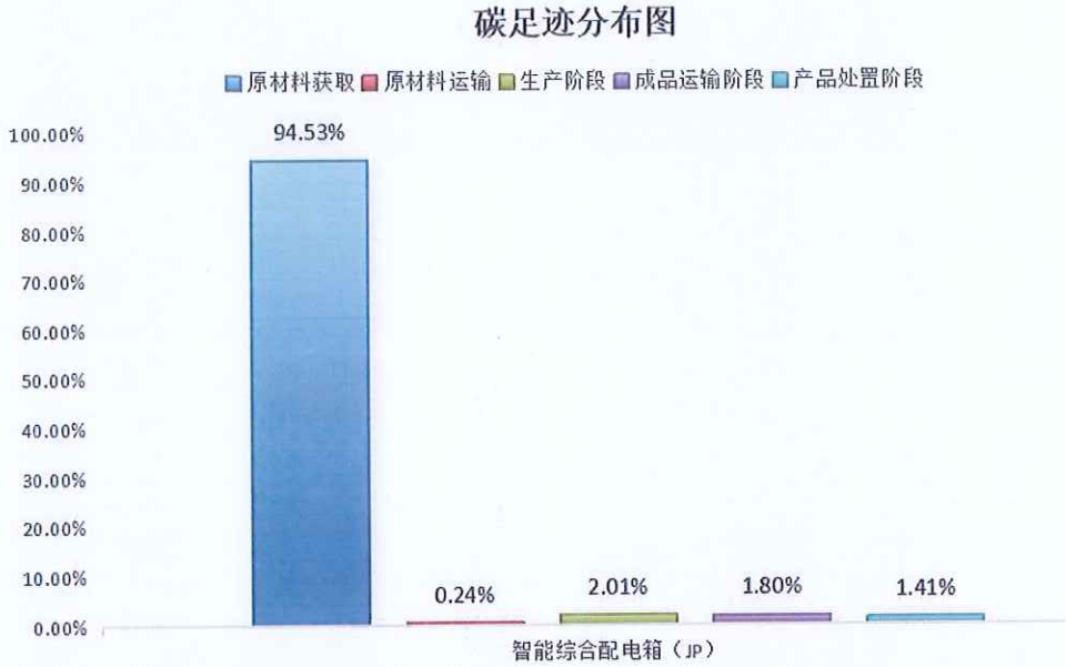
图 5.2-2 智能综合配电箱（JP）生命周期阶段碳排放分布图
