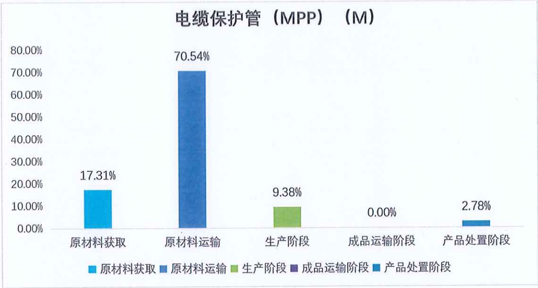
图 5.2-2 电缆保护管（MPP）生命周期阶段碳排放分布图
