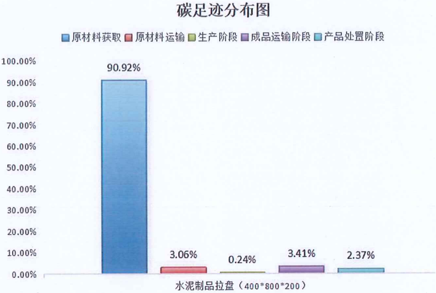
图 5. 2-2 水泥制品拉盘（400*800*200）生命周期阶段碳排放分布图
