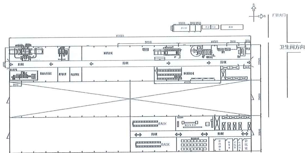
厂区布局图
