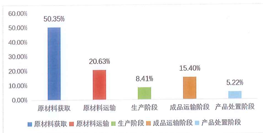
图 5.2.2-2 配电箱 JP、电缆分支箱 DFW 生命周期阶段碳排放分布图
