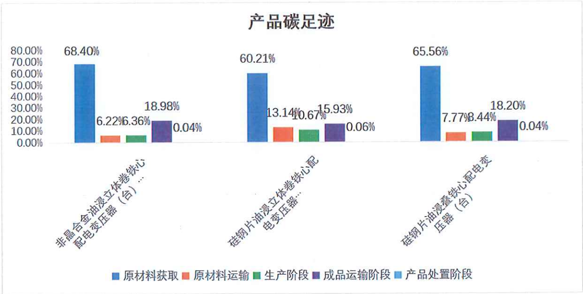
图 5.2.4 变压器生命周期阶段碳排放分布图
