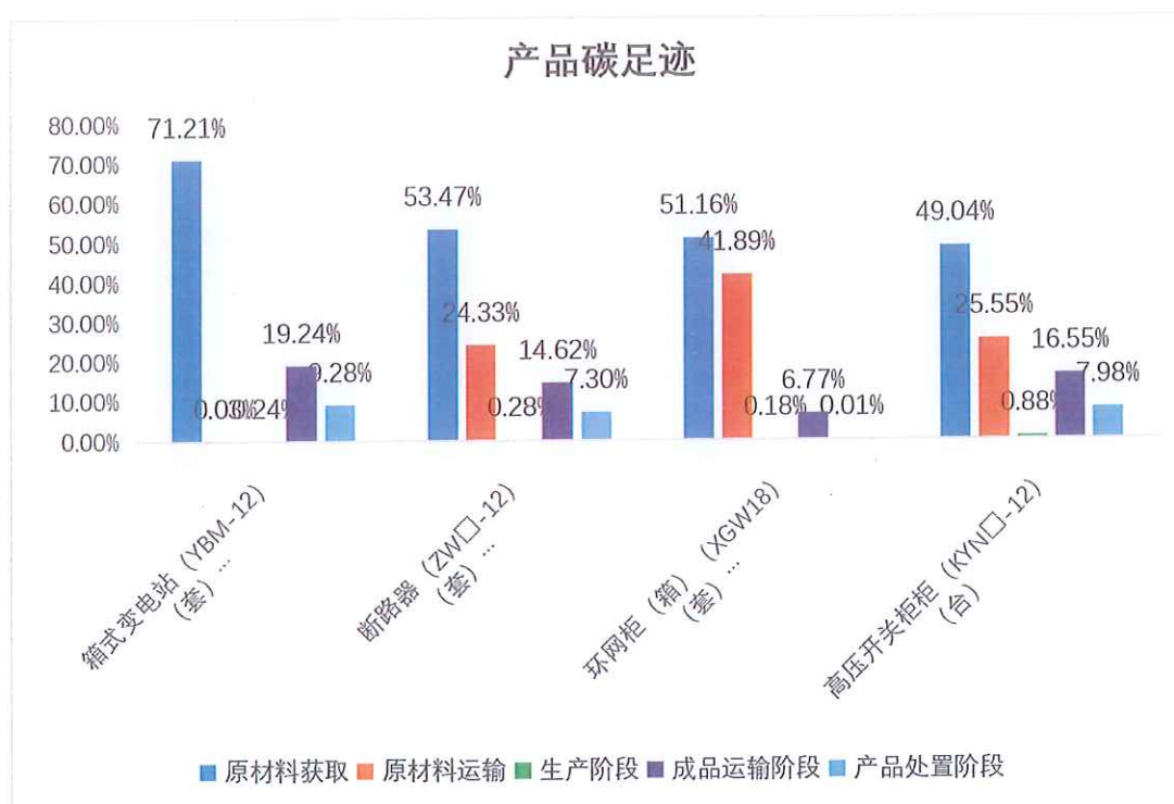
图 5.2.5 箱式变电站 (YBM-12) 断路器 (ZW□-12)、环网柜 (箱) (XGW18)、高压开关柜 (KYN□-12) 生命周期阶段碳排放分布图
