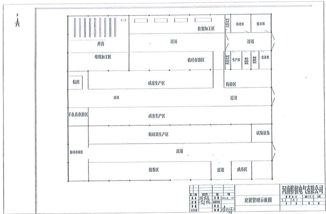
线束车间布局
