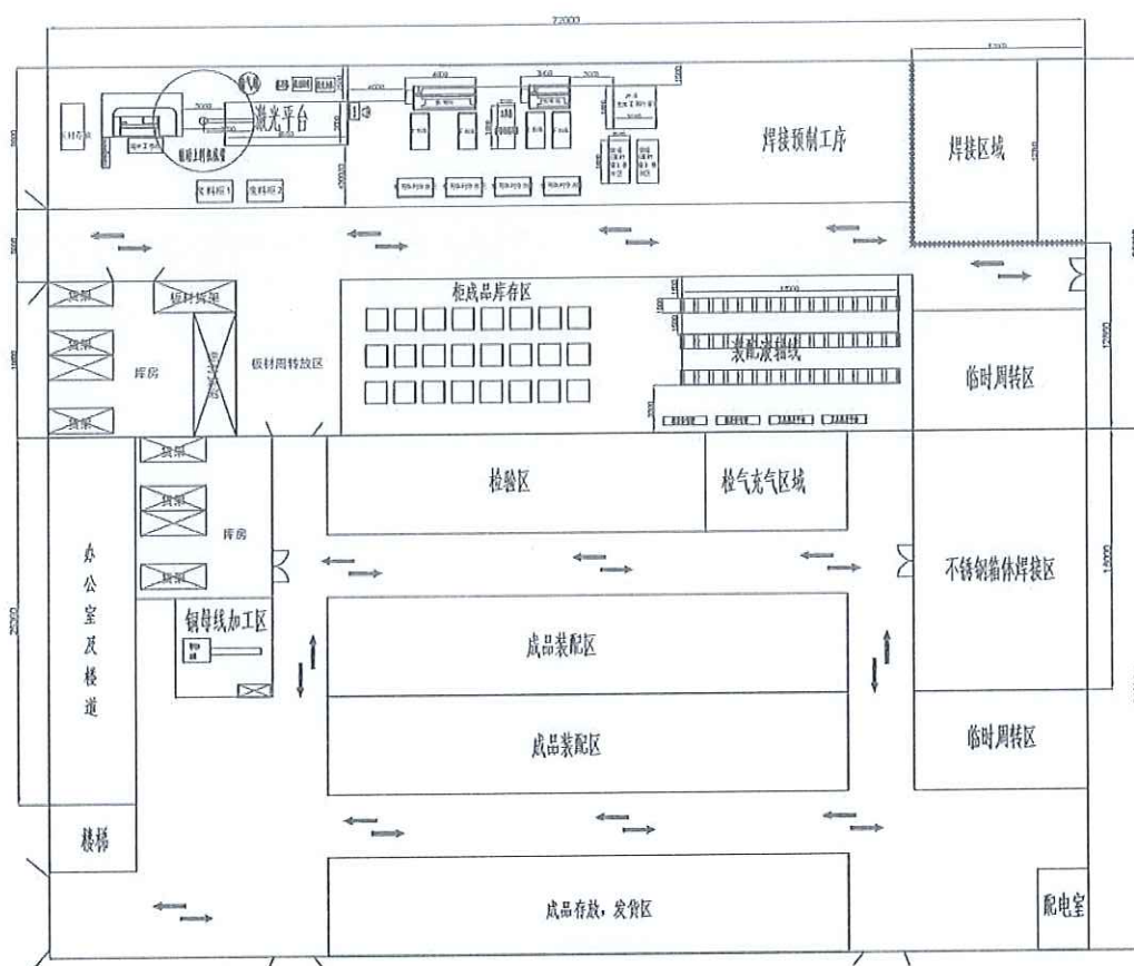
生产布局图
