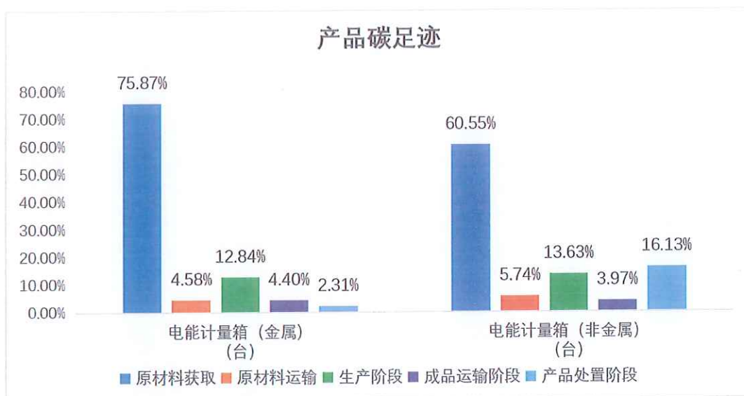
图 5.2.3 电能计量箱（金属、非金属）生命周期阶段碳排放分布图
