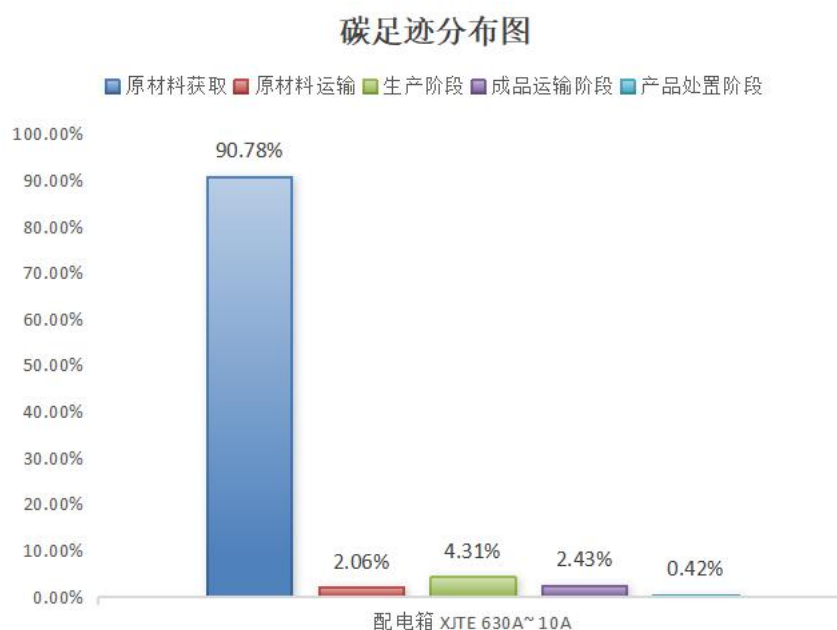
图 5.2-2 配电箱 XJTE 630A~ 10A 生命周期阶段碳排放分布图
