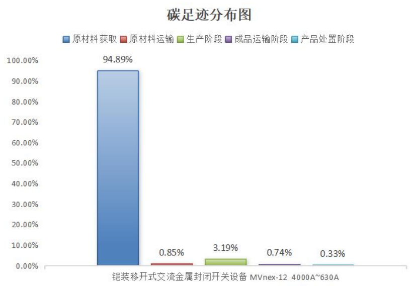
图 5.2-2 铠装移开式交流金属封闭开关设备 MVnex-12 4000A~630A 生命周期阶段碳排放分布图
