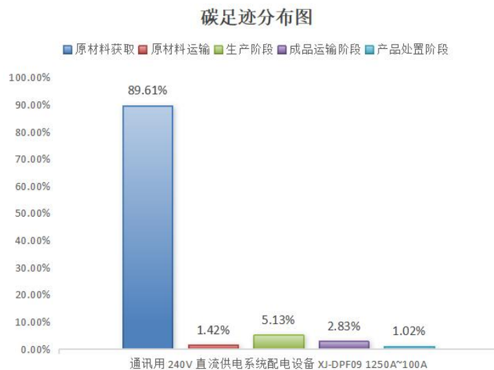
图 5.2-2 通讯用 240V 直流供电系统配电设备 XJ-DPF09 1250A~100A 生命周期阶段碳排放分布图
