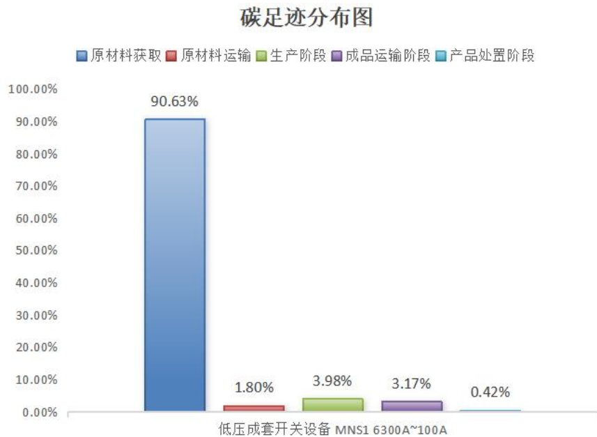
图 5.2-2 低压成套开关设备 MNS1 6300A~100A 生命周期阶段碳排放分布图
