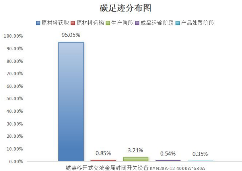
图 5.2-2 铠装移开式交流金属封闭开关设备 KYN28A-12 4000A~630A 生命周期阶段碳排放分布图
