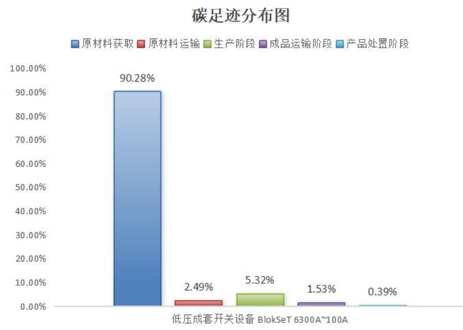
图 5.2-2 低压成套开关设备 BlokSeT 6300A~100A 生命周期阶段碳排放分布图
