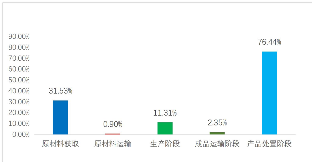
图 5.2.2 卧式母线系统（IHBS-D 1600A~250A）生命周期阶段碳排放分布图
