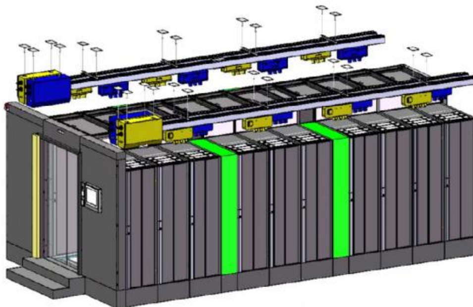
数据机房末端母线槽（MMS 800A~100A）
