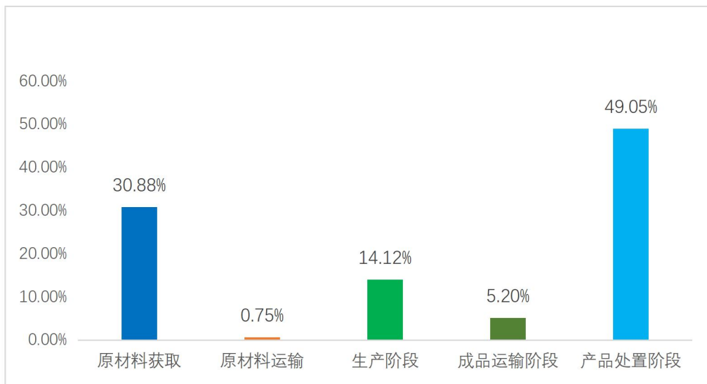
图 5.2.2 数据机房末端母线槽（MGS 630A~100A）生命周期阶段碳排放分布图
