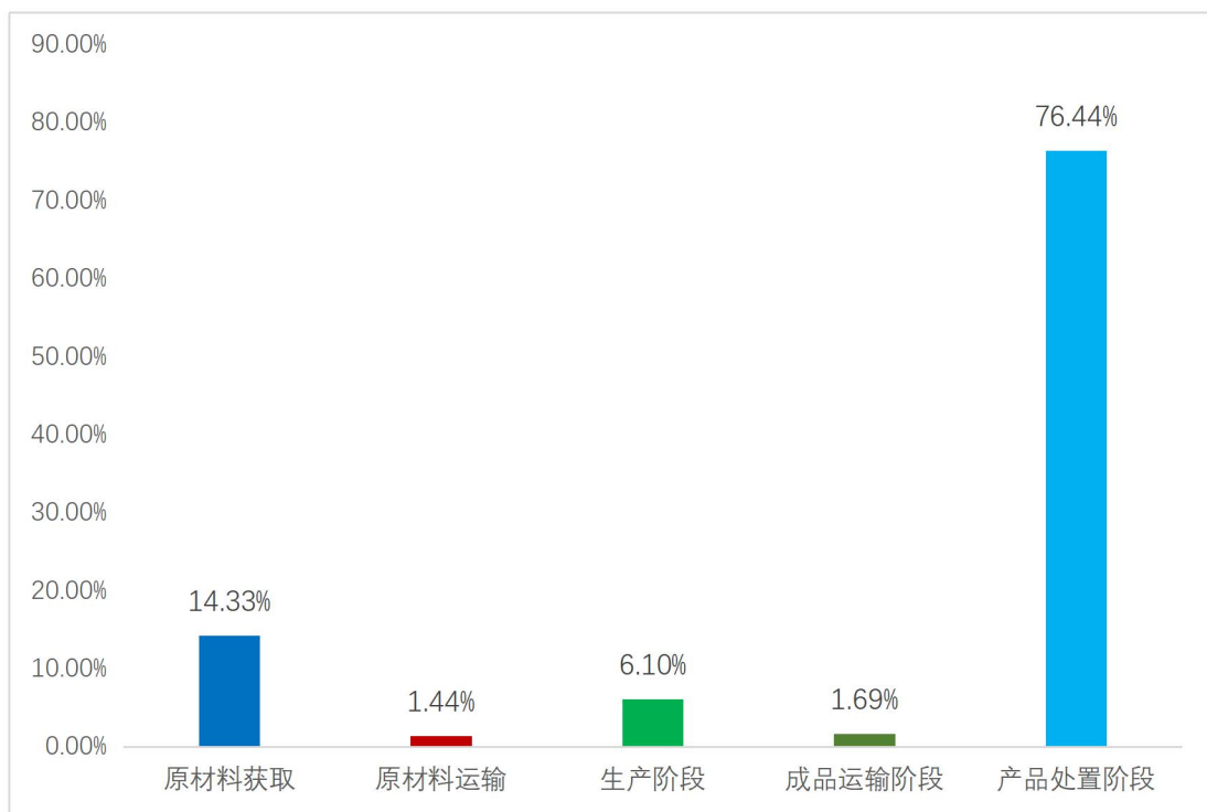
图 5.2.6-2 密集型母线槽（BMC10 6300A~400A）生命周期阶段碳排放分布图
