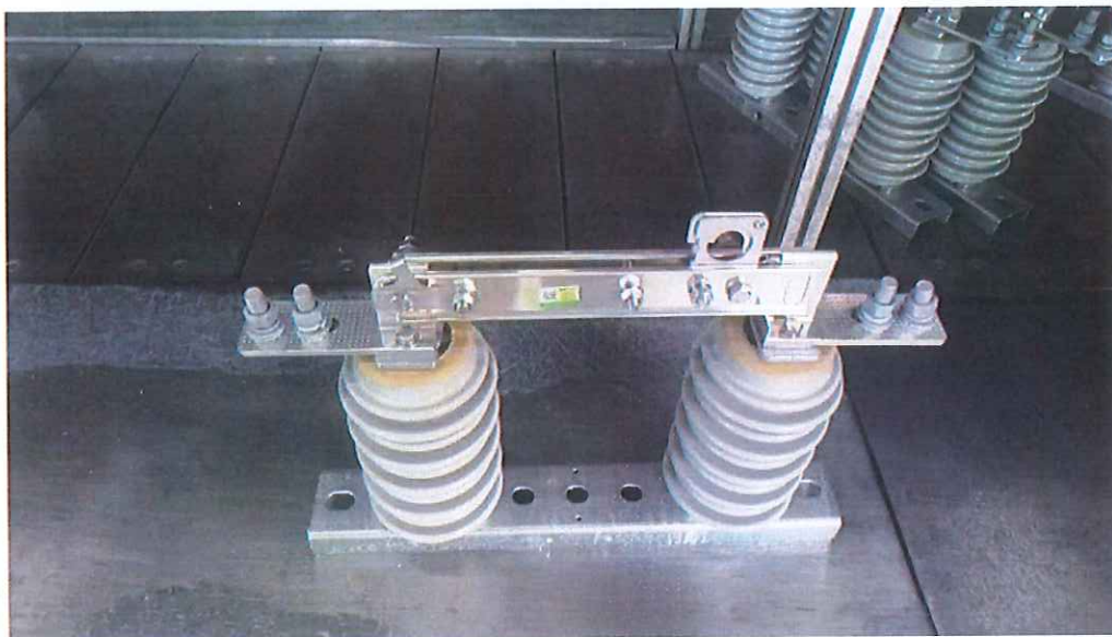
交流隔离开关（GW9-12GW/630-20）
