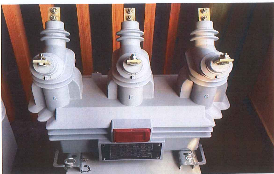
互感器 (JZZV1-10)
