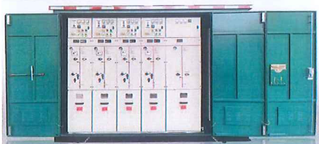
一二次融合成套环网箱（DGHBN-12(V、C、PT) / 630-20、KE-7120-B）
